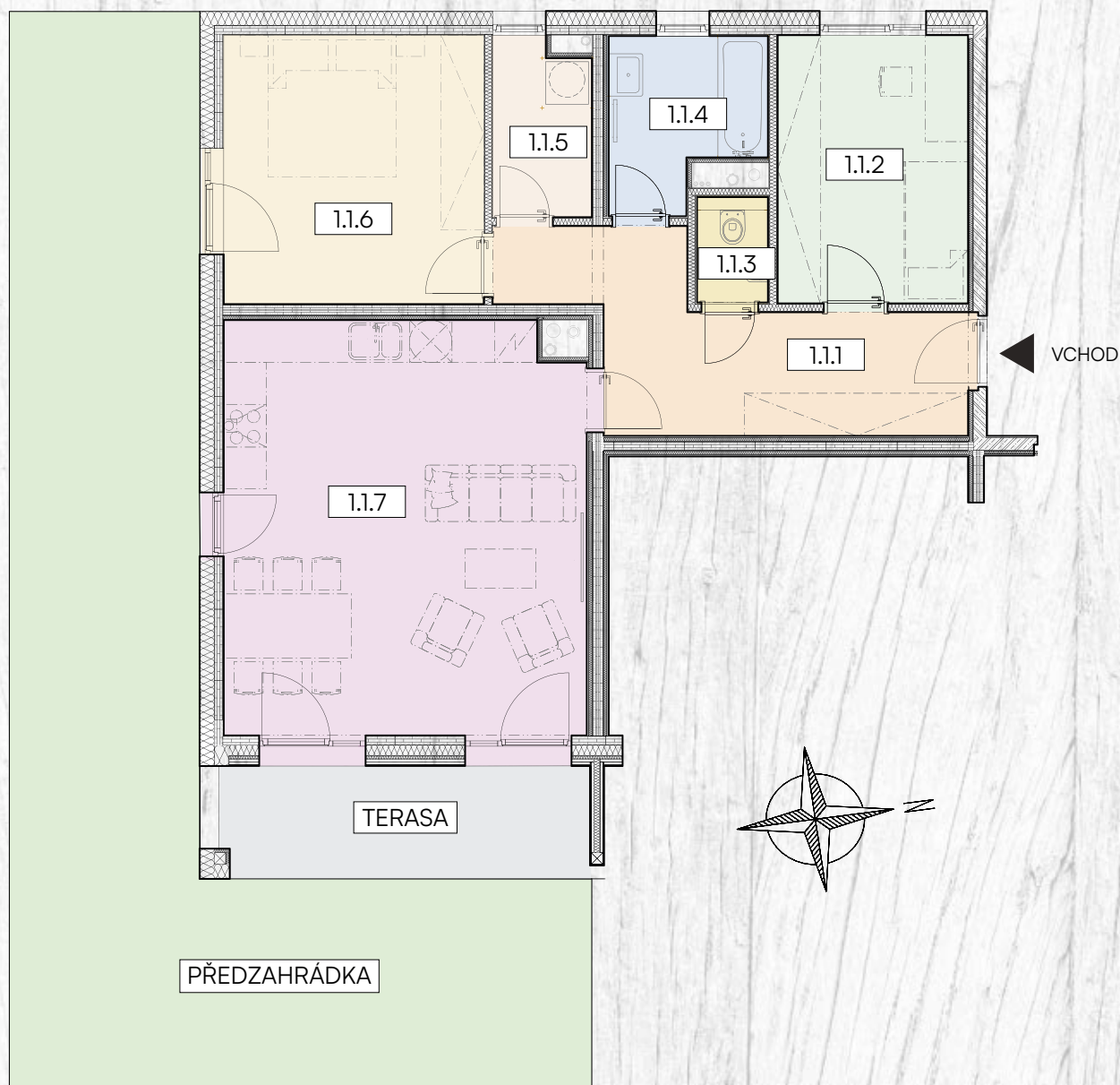
PŮDORYS BYTU
